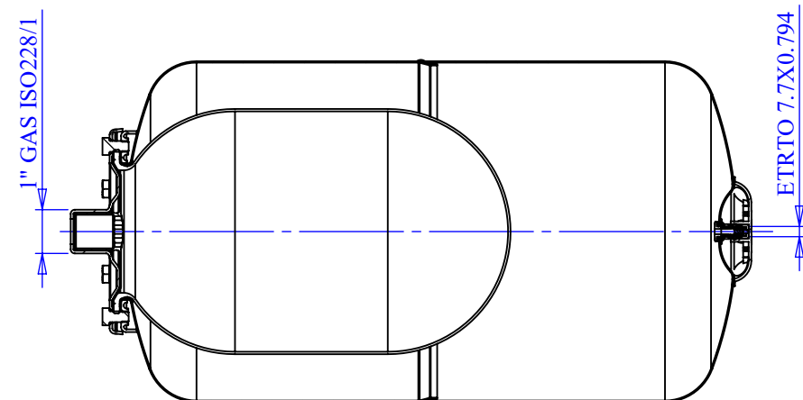
SEZIONE A-A
